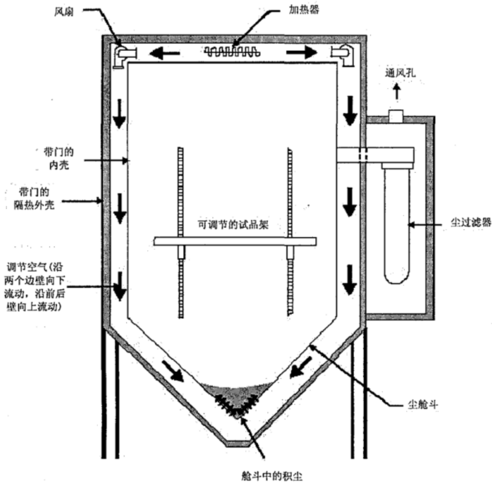
图1 降尘试验装置示例
